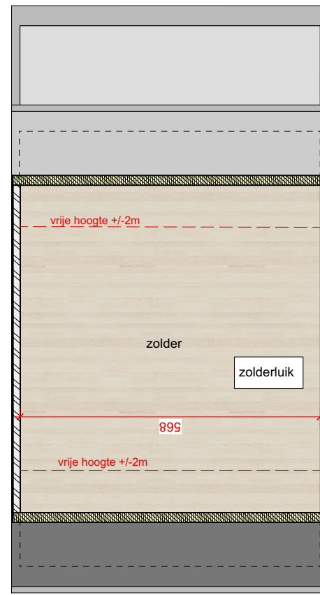
2e verdiep
