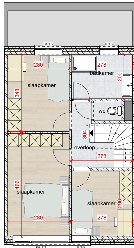
1e verdiep
